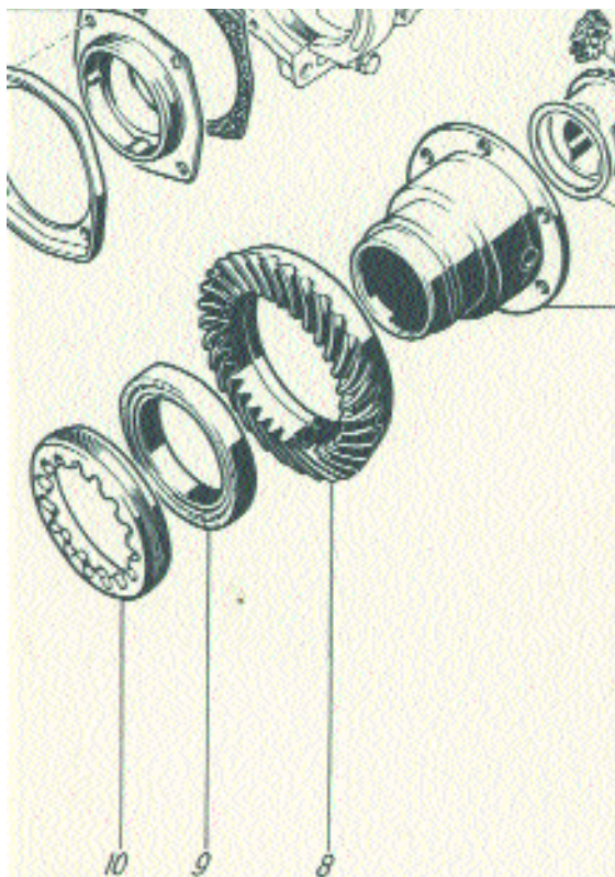
Abbildung 2: Differentialrad
