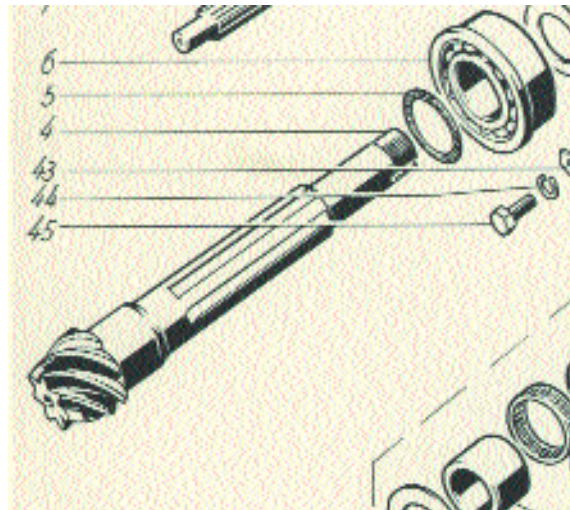
Abbildung 1: Abtriebswelle
