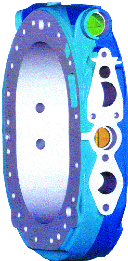
Bild 1: Vorderansicht Trochoide
